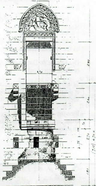
Vue en élévation des parties architecturales in situ mises au jour au cours du sondage (dessin de VIOLLET LE DUC).
